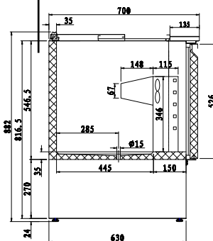
SALADETTE TOP 2P
