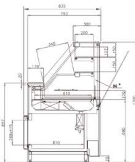
ELITE SLIM Avec réserve réfrigérée RT
