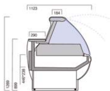
Version Bain-marie et salade pour bacs GN
