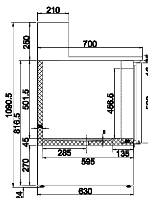
PIZZA TOP 2P
