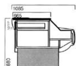
Meuble caisse avec repose sac et tiroir
