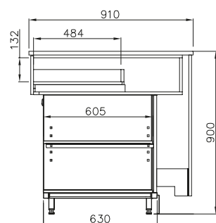
EVOLUCIA meuble caisse
