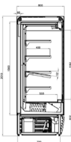
NAXOS STORE profondeur 800mm
