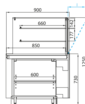
EVOLUCIA tourelle viennoiserie
