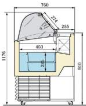
ANTILLE 4 LX sans réserve réfrigérée
