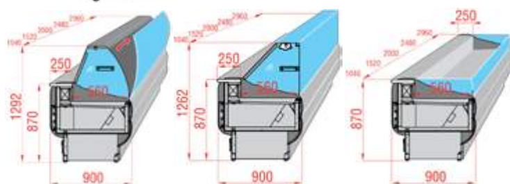
Vitrage courbe basculant
