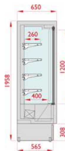
Ecoprima Slim avec portes Profondeur 650
