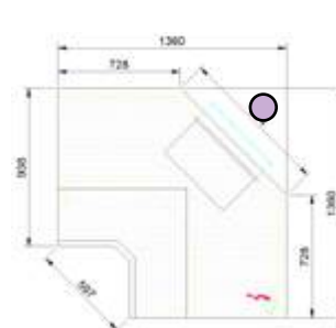
Caisse intérieur 90° long PMR
