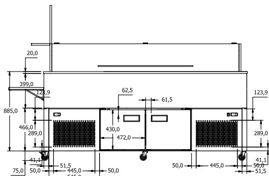
ATOLL BAR ALPHA 6
