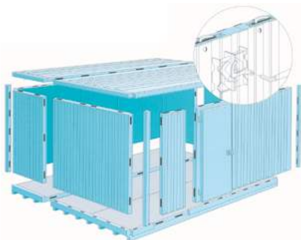
Assemblage des panneaux par crochets
