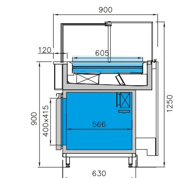
EVOLUCIA réfrigérée avec réserve vitrage haut
