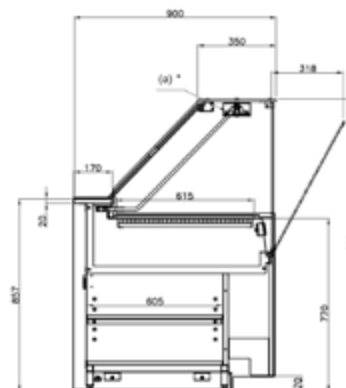
ELNTA plateau chaud vitrocéramique
