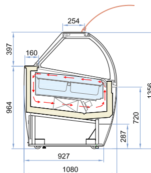
EQUATEUR B vitrage courbe
