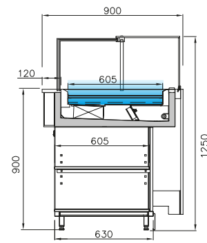
EVOLUCIA chocolat vitrage haut
