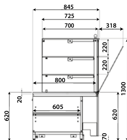
ELTV - Tourelle viennoiserie
