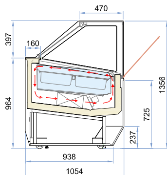
EQUATEUR D vitrage droit
