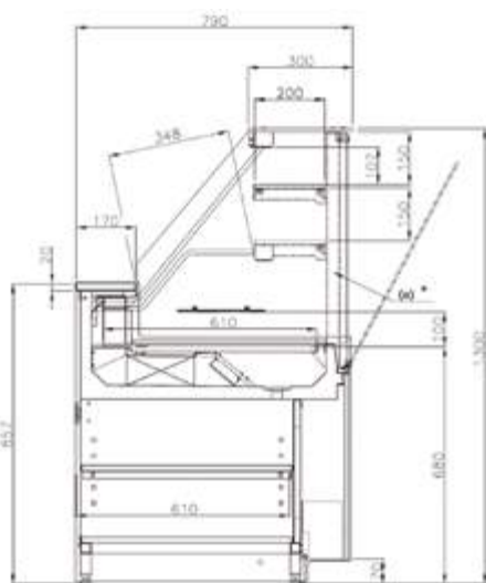
ELITE SLIM Sans réserve réfrigérée RS
