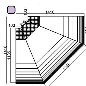
Angle ext. 90° Vitrage bombé VB
