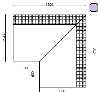
Angle droit int. 90° Vitrage droit VD
