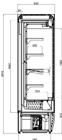
NAXOS Store Slim profondeur 620mm
