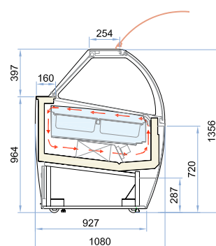
EQUATEUR B vitrage courbe
