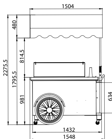
MINI DOLCE VITA
