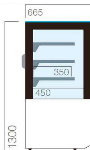
Version profondeur 665 mm
