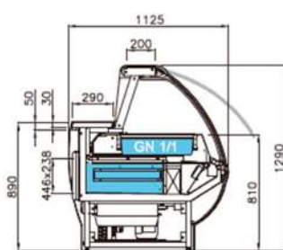
Version Bain-marie et salade pour bacs GN
