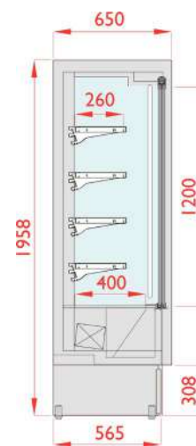
ECOPRIMA Slim avec portes Profondeur 650
