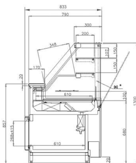
ELITE SLIM Avec réserve réfrigérée RT
