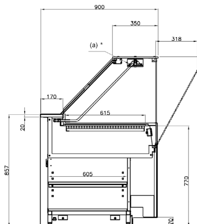
ELNTA plateau chaud vitrocéramique
