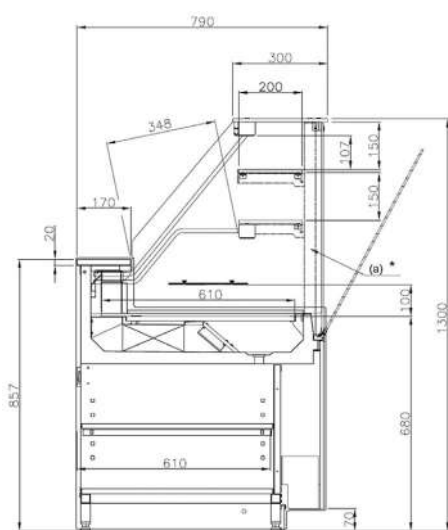
ELITE SLIM Sans réserve réfrigérée RS
