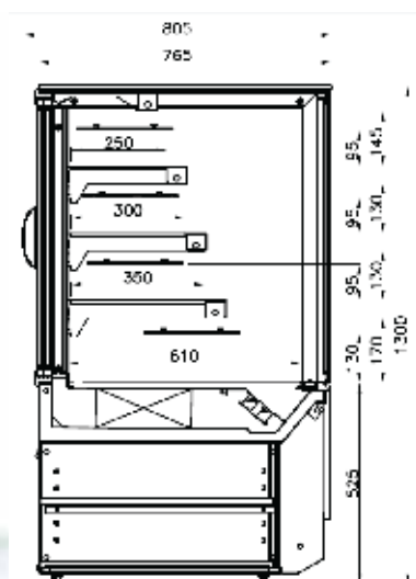
LUMIA - VITRE DROITE VD
