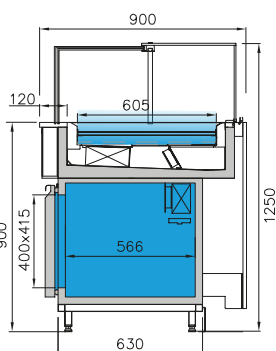
EVOLUCIA RÉFRIGÉRÉE AVEC RÉSERVE VITRAGE HAUT
