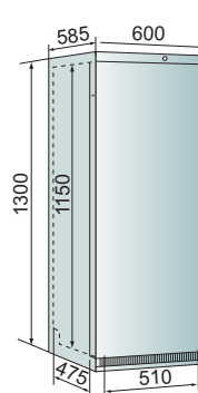
OLYMPUS 271 INOX VITRÉ
