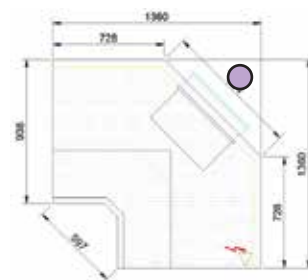
Caisse intérieur 90° long PMR
