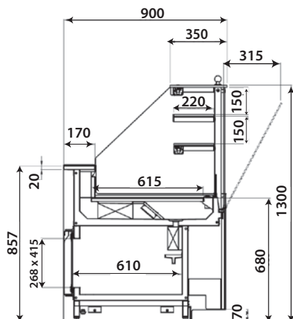
ELRTV Réfrigérée avec réserve
