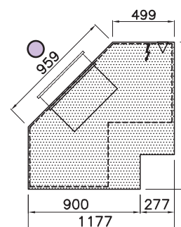
Meuble caisse Intérieur 90°
