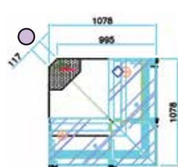
Angle ext. 90°
