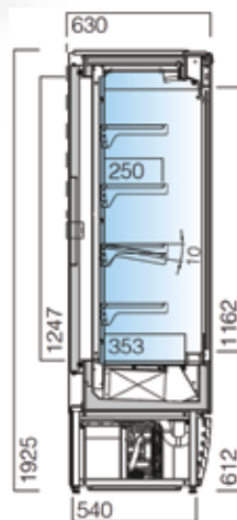
NAXOS SLIM INOX DOUBLE ACCÈS 190
