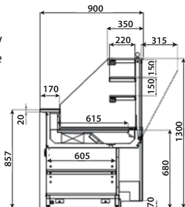
ELRSV Réfrigérée sans réserve
